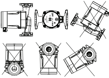
Fig. 2 Positions d'installation
