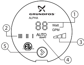
Fig. 7 Pantalla de control
